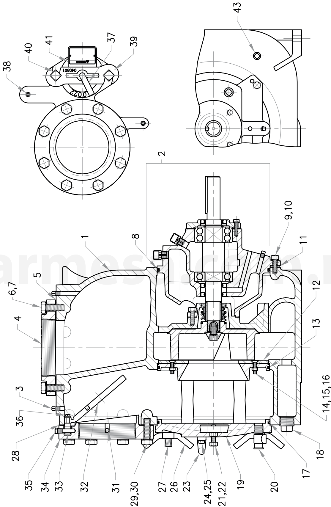
DIBUJO SECCIONAL DE BOMBA SH6-U
