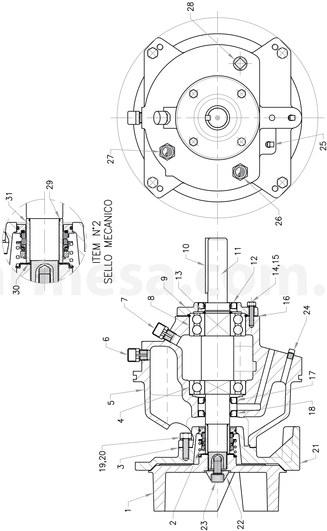
DIBUJO SECCIONAL DE EXTREMO MOTRIZ SH6-U
