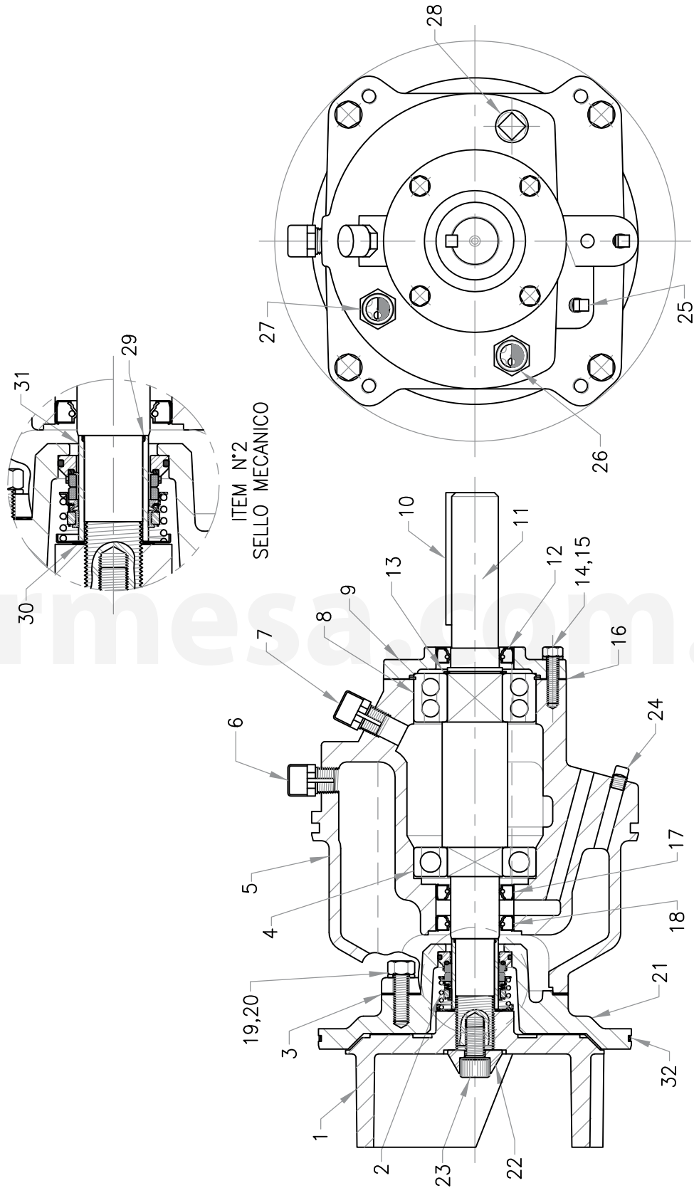
DIBUJO SECCIONAL DE EXTREMO MOTRIZ SH4
