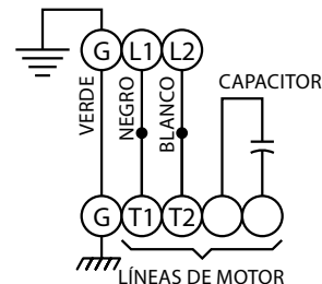
MONOFÁSICO 230V CA CABLE DE ALIMENTACIÓN 3x10
