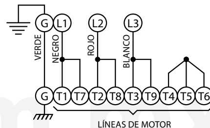
TRIFÁSICO 230V CA CABLE DE ALIMENTACIÓN 4x10
